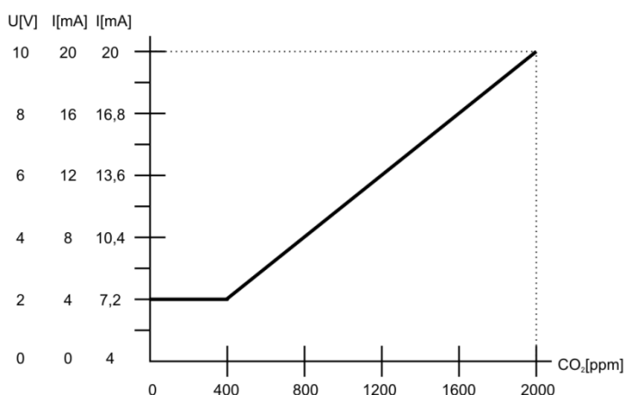
Graf závislosti výstupního napětí/proudu na koncentraci CO 2
